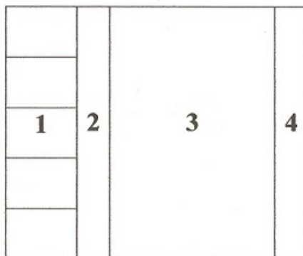
Рис. 1 Расчетная схема ограждающей конструкции: 1 – кирпичная кладка в \frac{1}{2} кирпича; 2 – воздушная прослойка; 3 – фибропенобетонный блок; 4 – гипсовая штукатурка.
